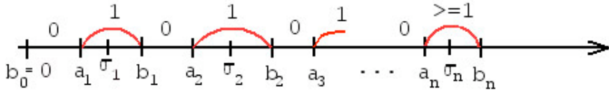
Abbildung 3.3.1: Darstellung der Zwischenankunftszeiten
