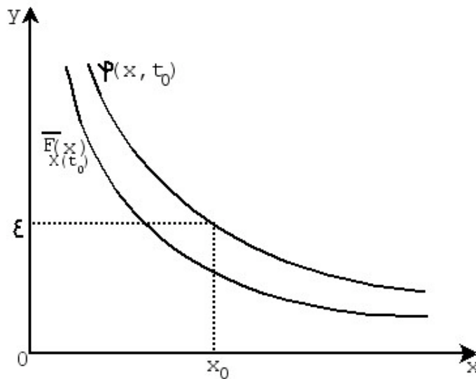
Abbildung 4.3.1: Darstellung von \varphi und \bar{F}_{X(t_0)}
