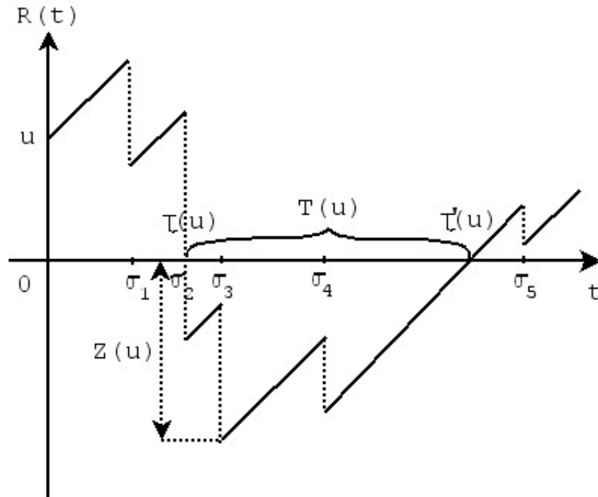
Abbildung 9.1.2: Darstellung eines Ruinprozesses
