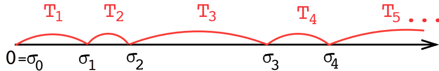
Abbildung 1.3.2: Schadenzeitpunkte \sigma_i und Zeitintervalle T_i
