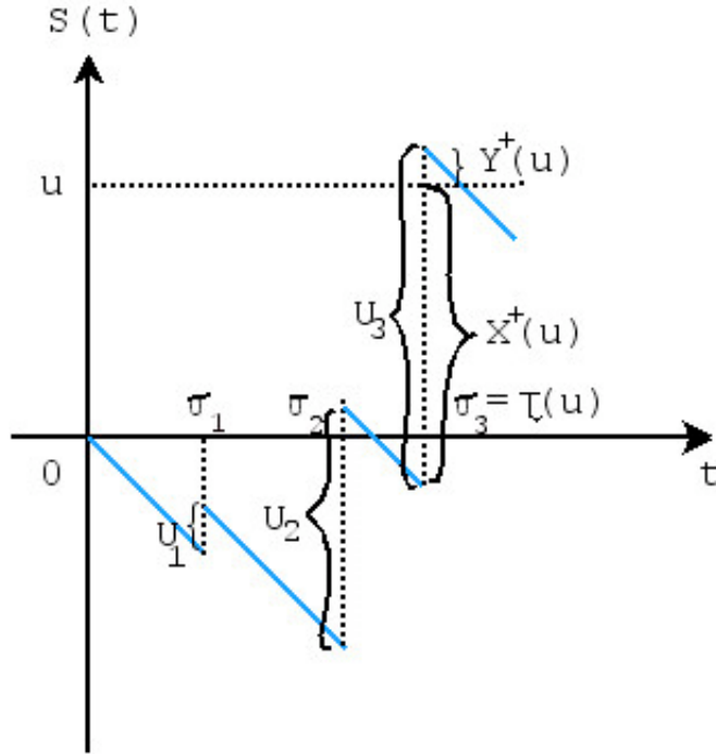
Abbildung 9.1.1: Darstellung eines Überschussprozesses
