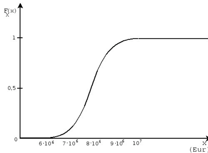
Abbildung 4.4.1: Verteilung des Gesamtschadens im Beispiel 4.4.2
