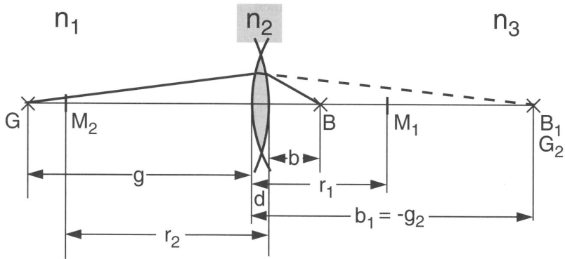
Bild 3.25: Abbildung durch eine dünne Linse. Für den Fall einer dünnen Linse (man kann die Linsendicke d gegenüber der Gegenstandsweite g , der Brennweite b und den Krümmungsradien der Linse vernachlässigen) gilt die einfache Abbildungsgleichung (3.27).
