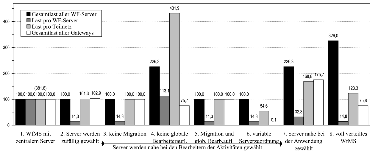
Abbildung 10 Ergebnis der Simulation II
