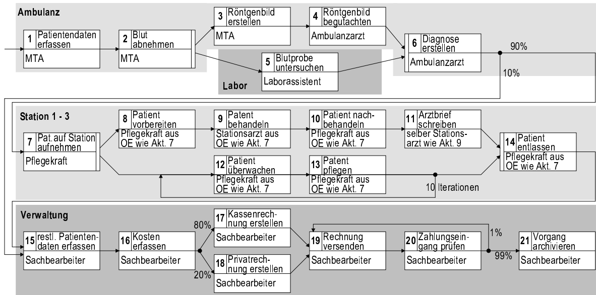
Abbildung 8 Für die Simulation verwendeter WF: Aktivitäten mit Bearbeiterzuordnung
