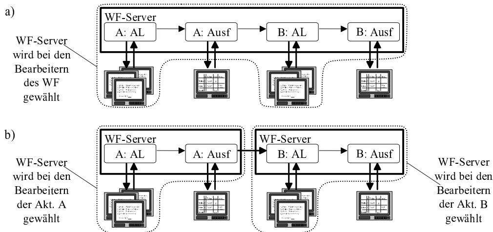
Abbildung 5 WF-Server nahe bei den potentiellen Bearbeitern, Granularität: a) gesamter Prozeß (ohne Migration), b) einzelne Aktivitäten (mit Migration)
