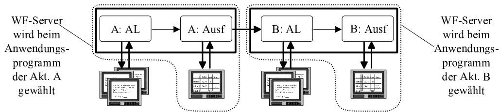
Abbildung 6 Der WF-Server wird nahe bei Anwendung plaziert
