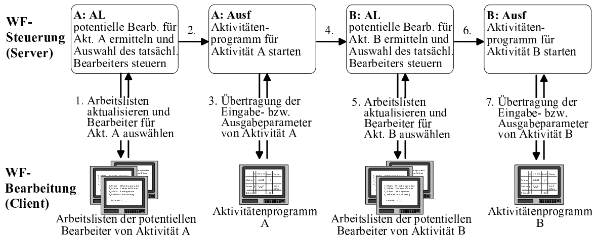
Abbildung 1 Steuerung und Bearbeitung eines WF, der aus den Aktivitäten A und B besteht
