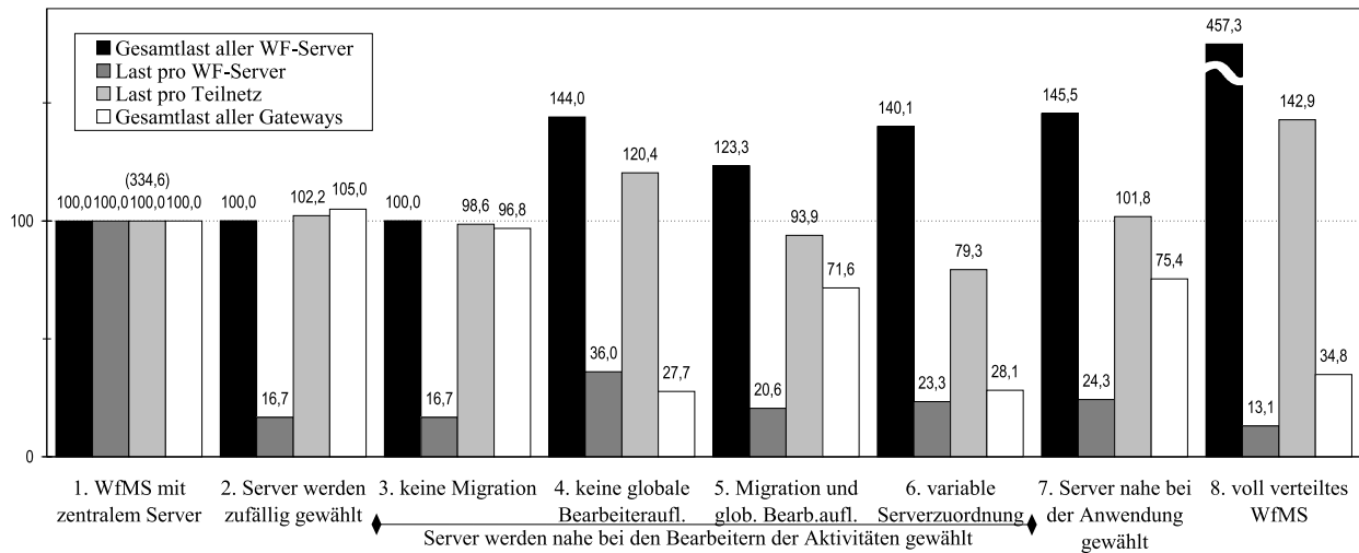
Abbildung 9 Ergebnis der Simulation I
