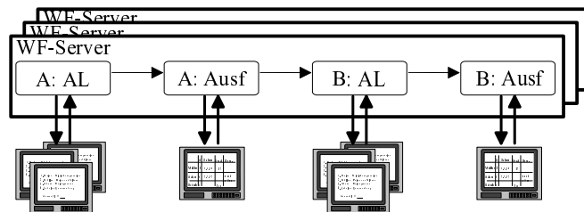
Abbildung 4 Der Cluster für eine WF-Instanz wird bei deren Start zufällig gewählt
