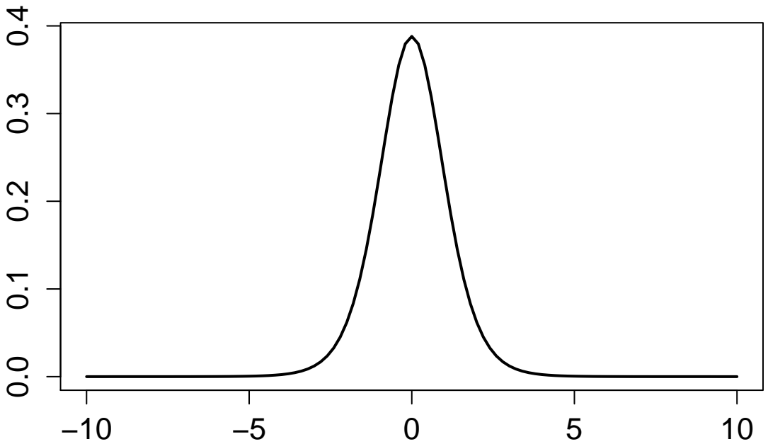
Dichte der t-Verteilung mit n = 9 Freiheitsgraden
