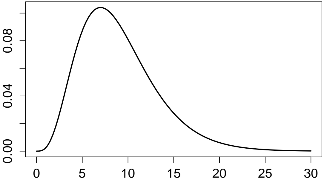
Dichte der \chi^2 -Verteilung mit n = 9 Freiheitsgraden
