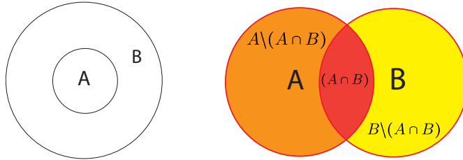
Abbildung 2.2: Illustration zu Satz 2.2.2, 3) und 4)
