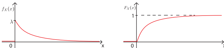
Abbildung 3.12: Dichte und Verteilungsfunktion der Exponentialverteilung \text{Exp}(\lambda) .
