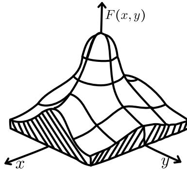
Abbildung 3.17: Grafik der Dichte einer zweidimensionalen Normalverteilung
