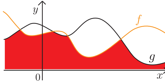
Abbildung 7.1: Illustration zur Ungleichung (7.8)
