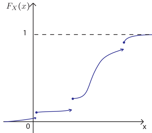
Abbildung 3.6: Typische Verteilungsfunktion
