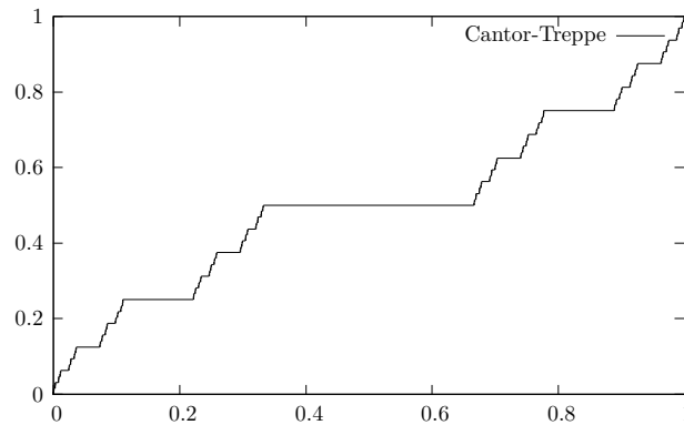
Abbildung 3.15: Cantor-Trepp
