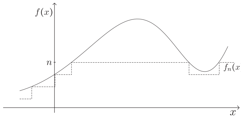
Abbildung 4.2: Approximation durch einfache Funktionen
