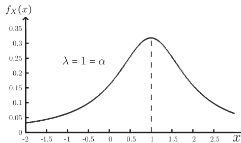
Abbildung 3.13: Dichte der \text{Cauchy}(\alpha, \lambda) -Verteilung
