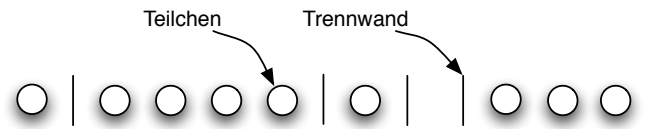
Abbildung 2.4: Ziehen ohne Reihenfolge und mit Zurücklegen
