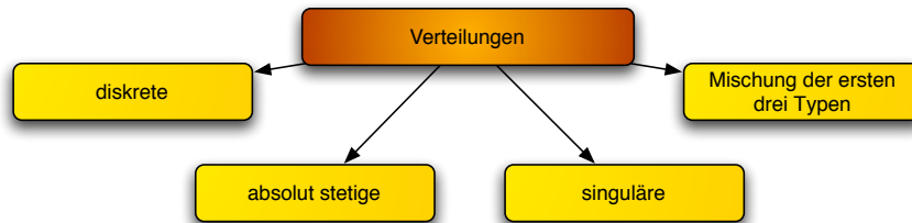
Abbildung 3.7: Verteilungstypen
