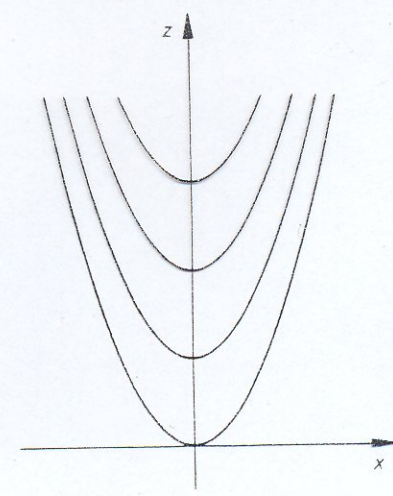
Bild IV-19 Schnittkurvendiagramm der Fläche z = x^2 + y^2 (Schnitte parallel zur x, z -Ebene)
