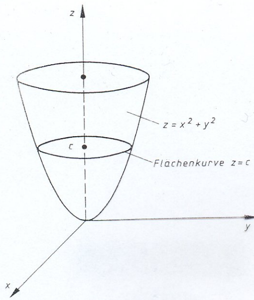
Bild IV-17 Schnitt der Fläche z = x^2 + y^2 mit der Parallelebene z = c
