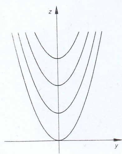
Bild IV-18 Schnittkurvendiagramm der Fläche z = x^2 + y^2 (Schnitte parallel zur y, z -Ebene)
