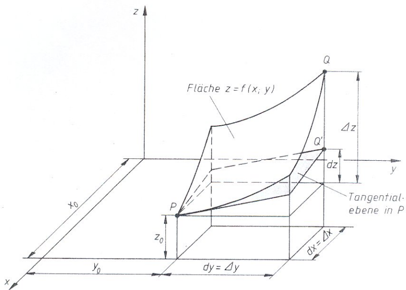
Bild IV-28 Zum Begriff des totalen oder vollständigen Differentials einer Funktion z = f(x, y)
