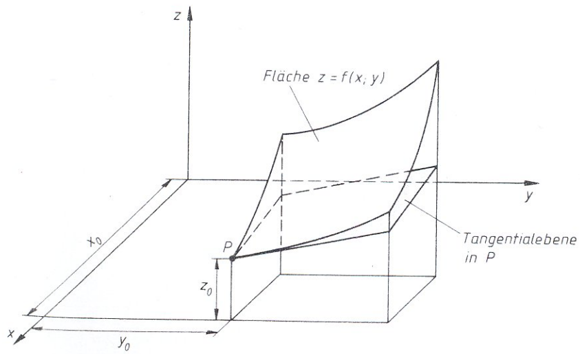
Bild IV-27 Tangentialebene an die Fläche z = f(x, y) im Flächenpunkt P = (x_0; y_0; z_0)
