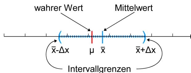
Abbildung 2: Fehlerintervall
