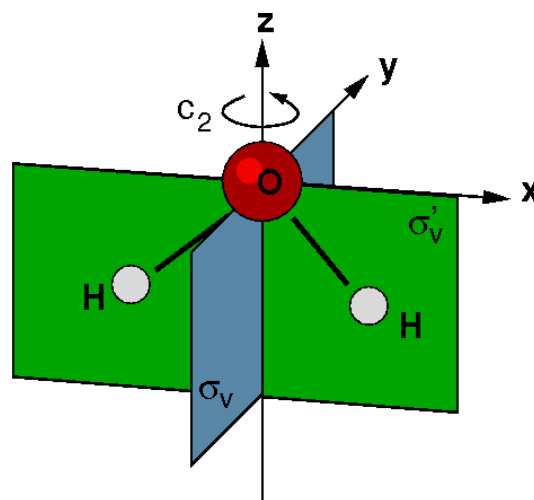
Abbildung 1: Das H 2 O Molekül und seine Symmetrieeoperationen.
