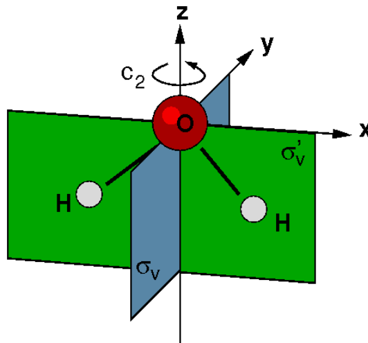
Abbildung 1: Das H_2O Molekül und seine Symmetrieoperationen.
